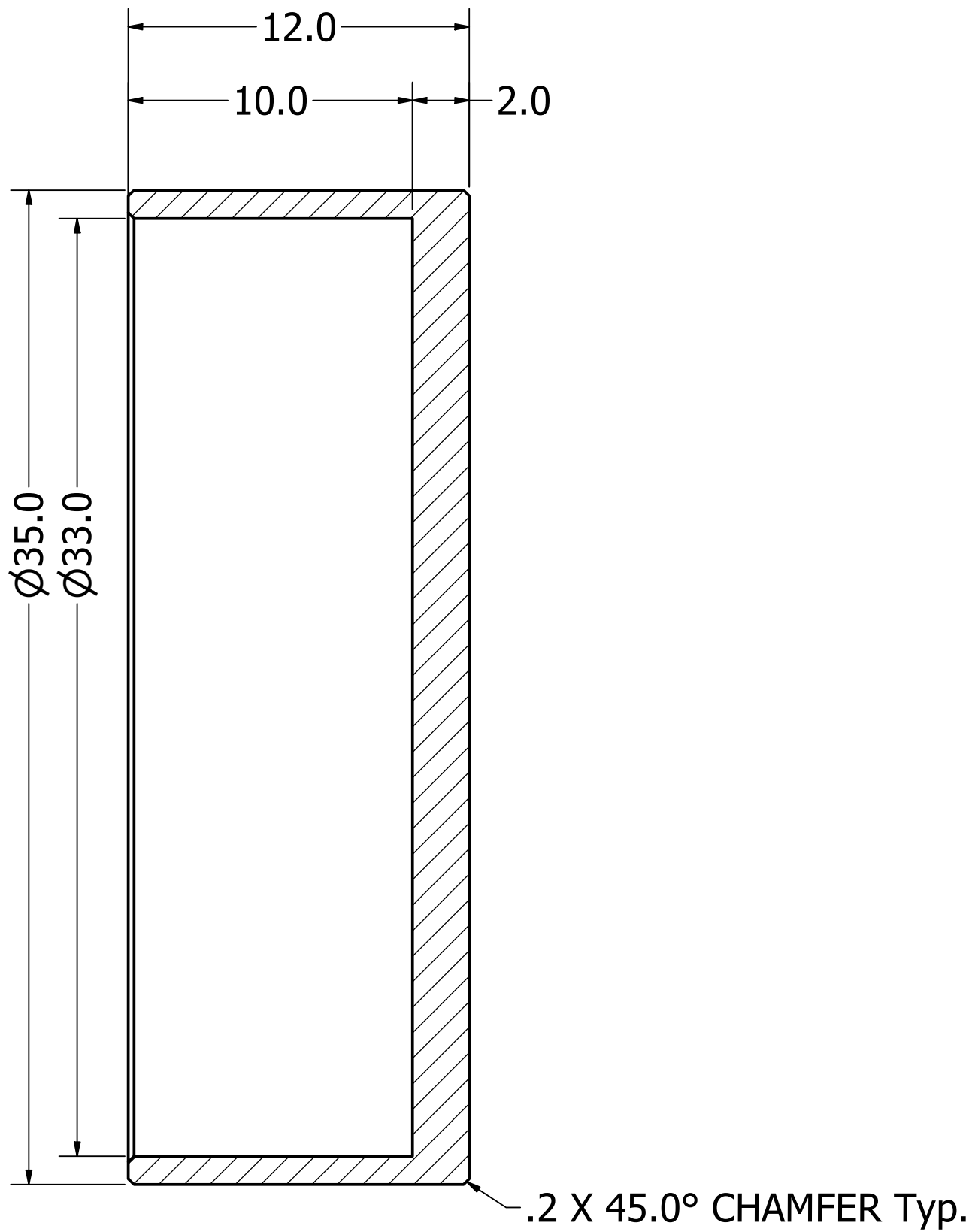
SECTION A-A SCALE 5 : 1
